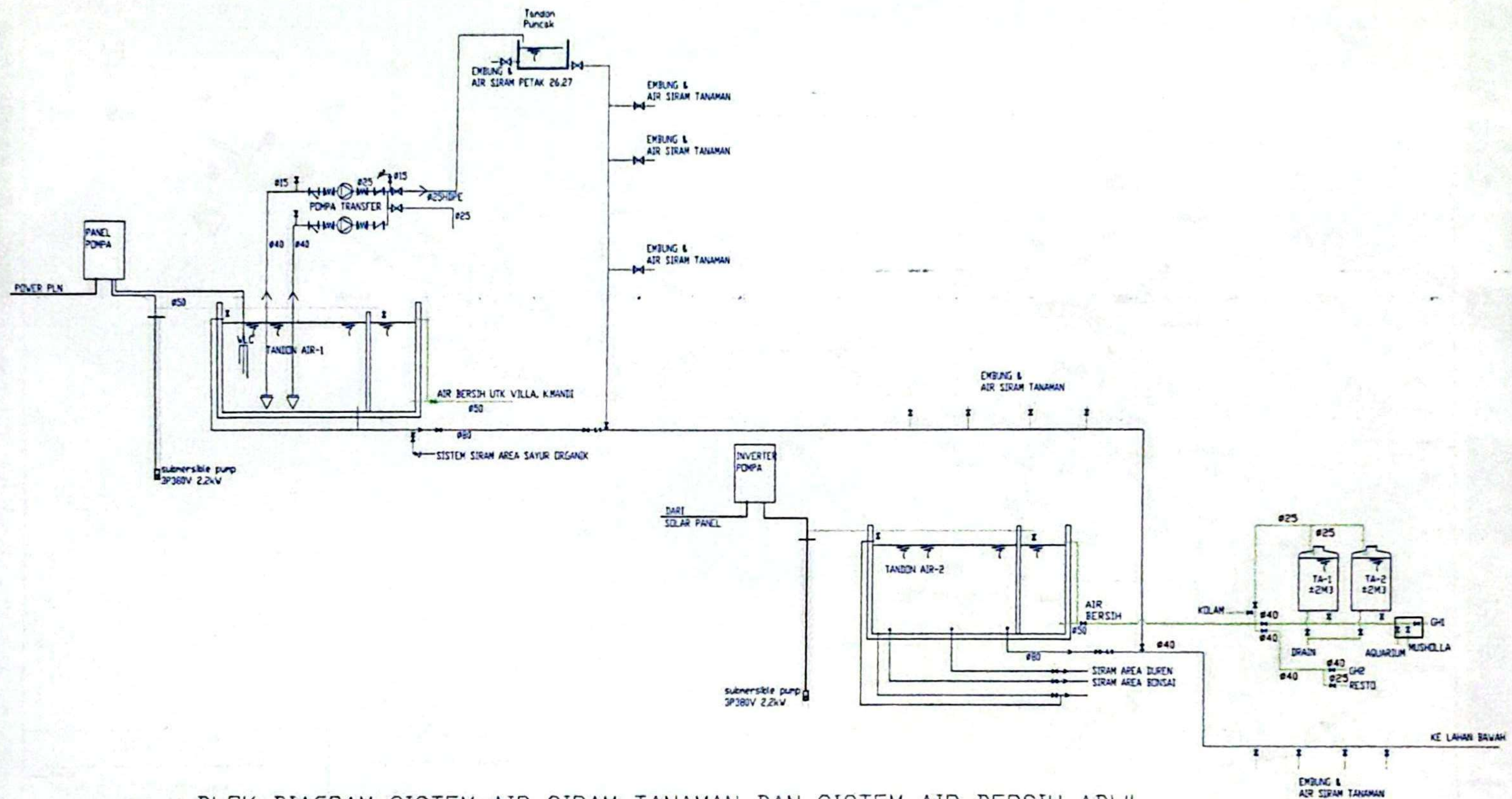
BLOK DIAGRAM SISTEM AIR SIRAM TANAMAN DAN SISTEM AIR BERSIH ABWL
